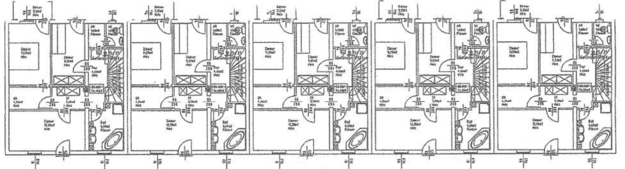
Obergeschoss
