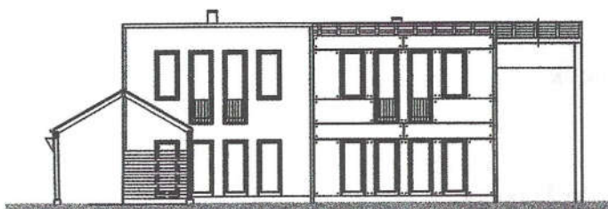
ANSICHT SÜD
