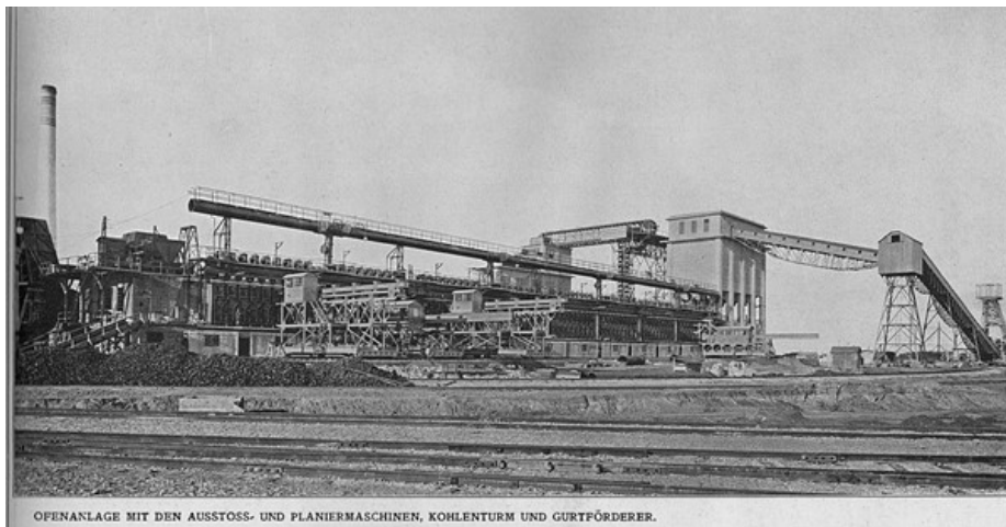
ABBILDUNG 2: STÄDTISCHE GASWERK LEOPOLDAU: OFENANLAGE MIT DEN AUSSTOSS- UND PLANIERMASCHINEN, KOHLENTURM UND GURTFÖRDERER, 1911, AUTOR/URHEBER: CHWALA'S DRUCK UND VERLAG, WIEN 7 2
